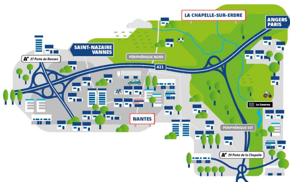
Aménagement de la Porte de Gesvres entre la Porte de La Chapelle (n°39) et la Porte de Rennes (n°37)
